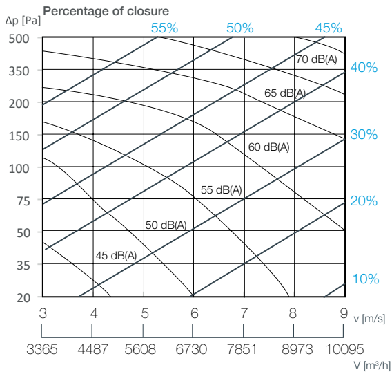
Ød630
