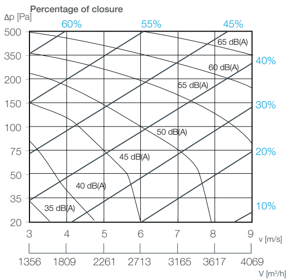
Ød630
